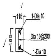
LINTEL BEAM-2
