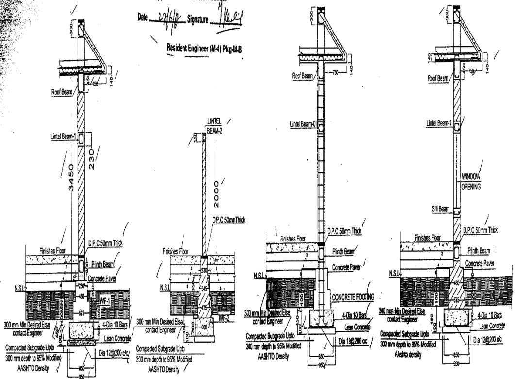
SECTION D-D
