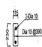
DOOR JAMB
